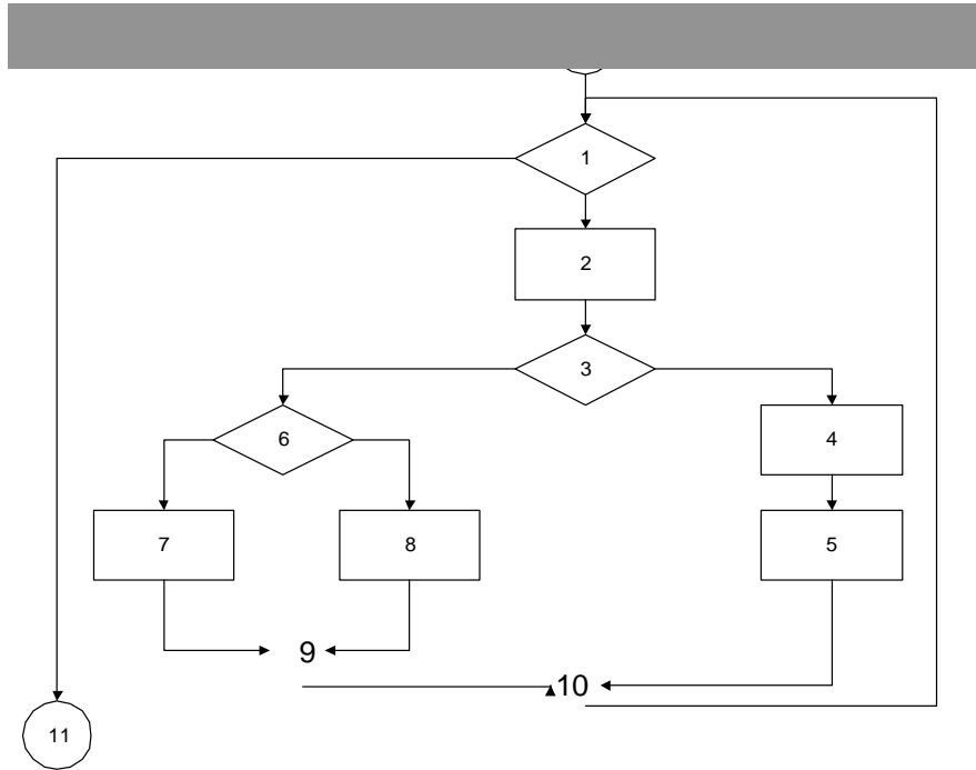
Gambar 9.2 Diagram Alir
