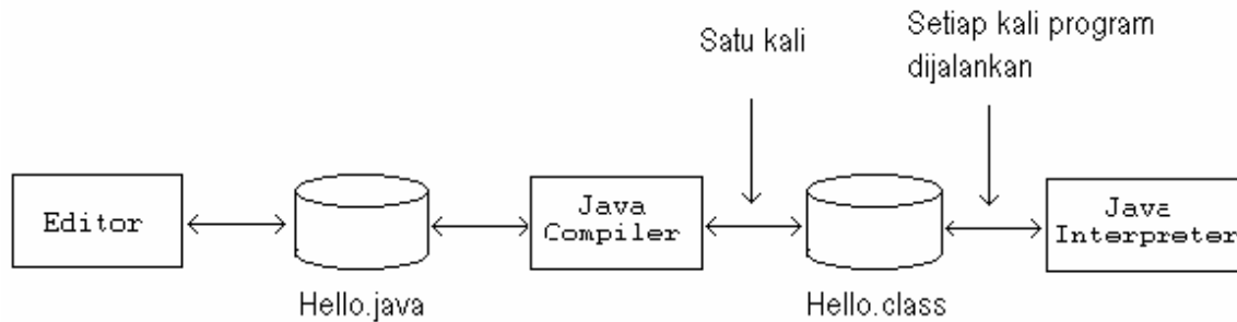
Gambar 2.1: Fase dari sebuah Program Java
